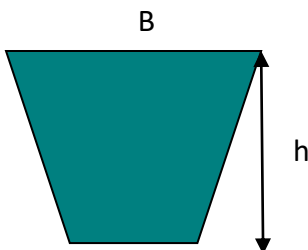
Trapezio
