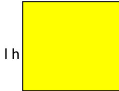
Cuadrado
