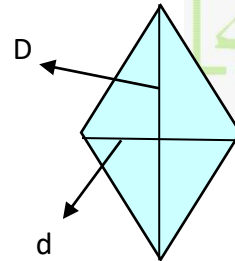
Rombo
