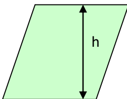
Paralelogramo
