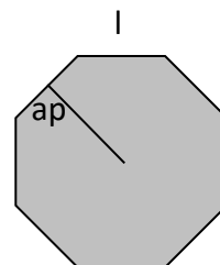
Polígonos Regulares
